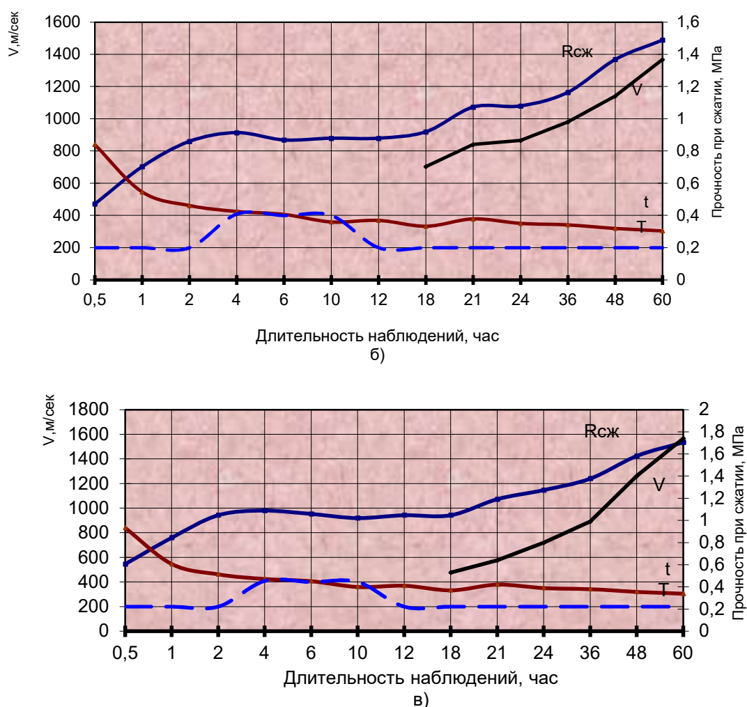
Рисунок 1 - Кривые кинетики структурообразования шлакощелочного арболита на древесной дробленке (ДД). а – вяжущее + ДД; б – то же, + 3ШС; в – то же, +3ШС + ХСДБ (хромпик).
